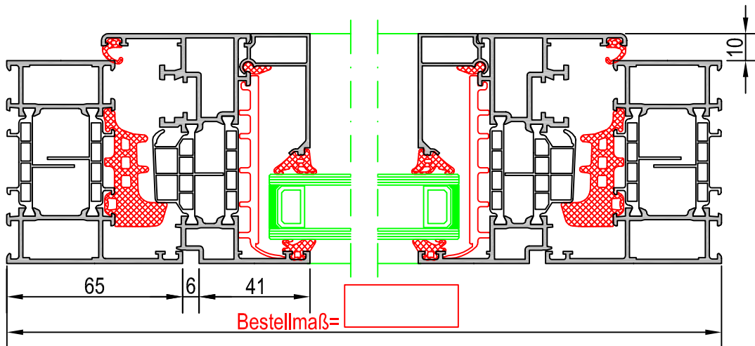
Horizontalschnitt M 1:2
