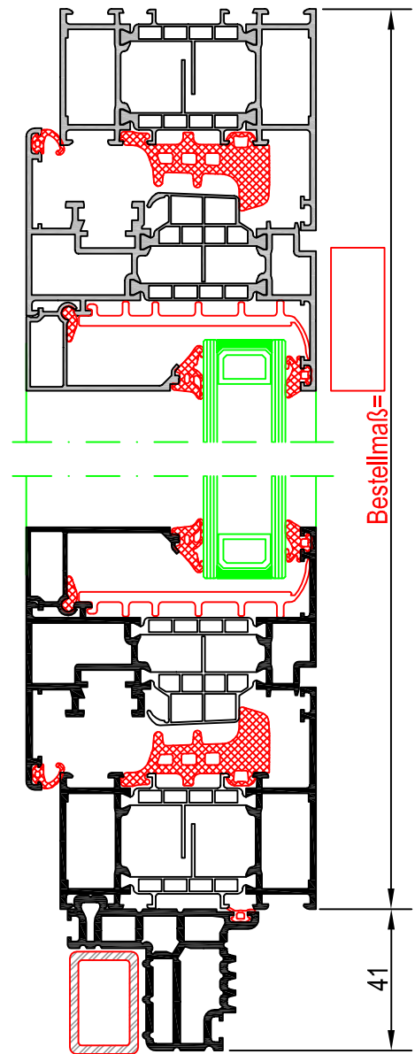
Vertikalschnitt M 1:2
